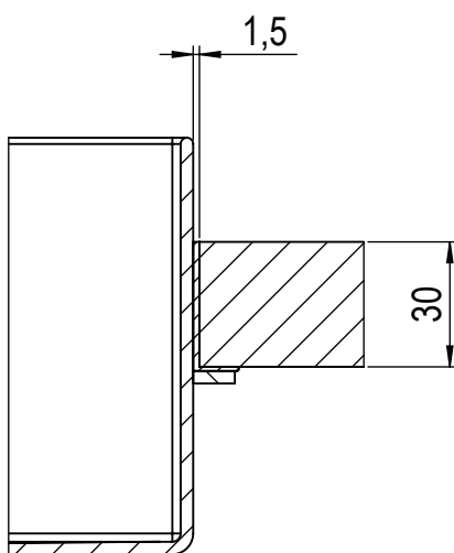
A-A (1 : 2)
