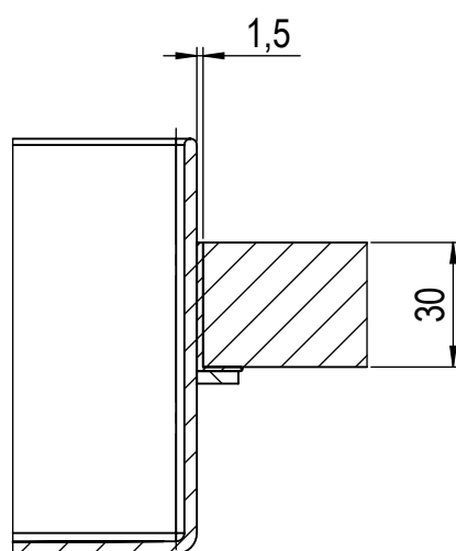
A-A (1 : 2)
